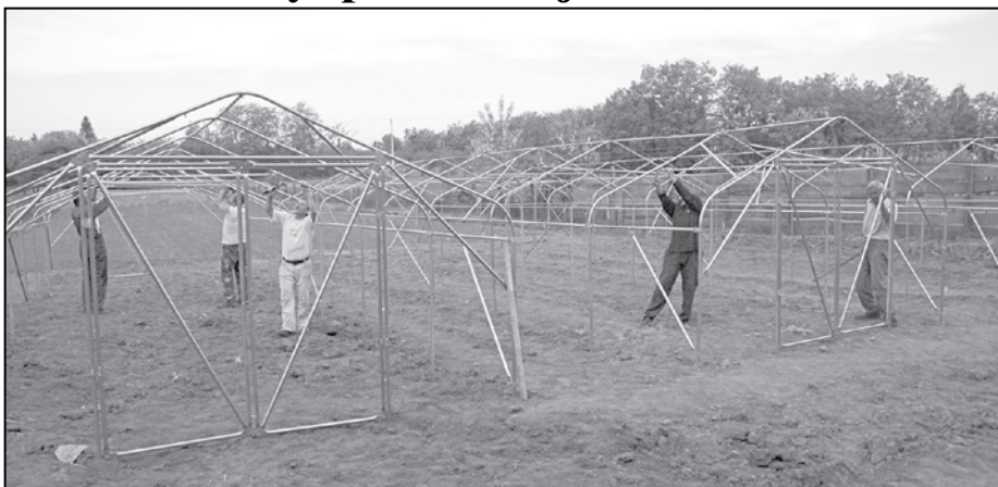
Így épült a fóliaház
